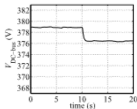
Fig. 17. Case A: dc bus voltage profile.
